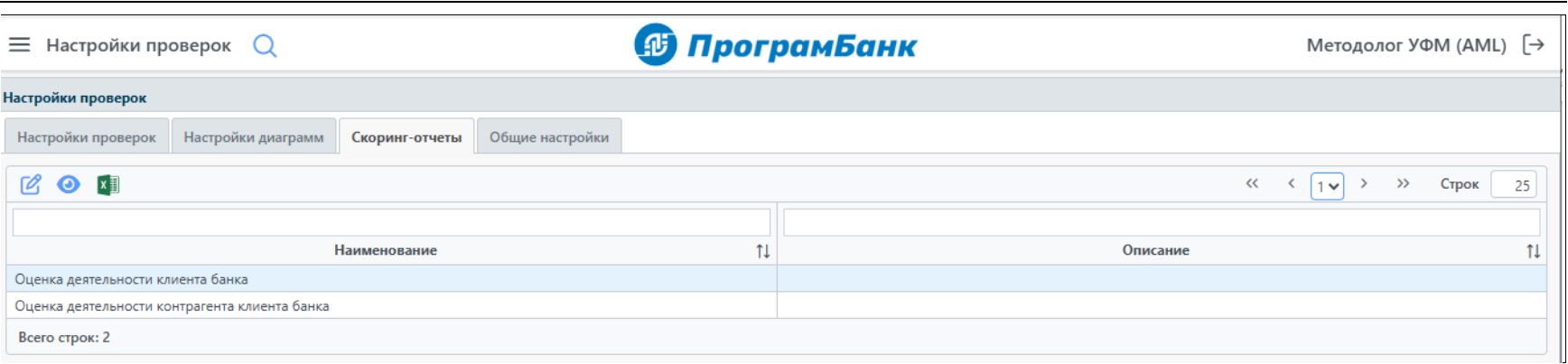
рисунок 49. Вкладка "Скоринг-отчеты"
