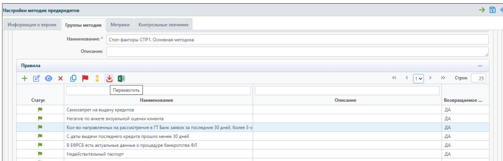
рисунок 13. Перемещение правил
