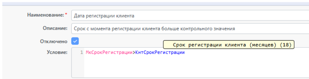
рисунок 14. Параметры правила
